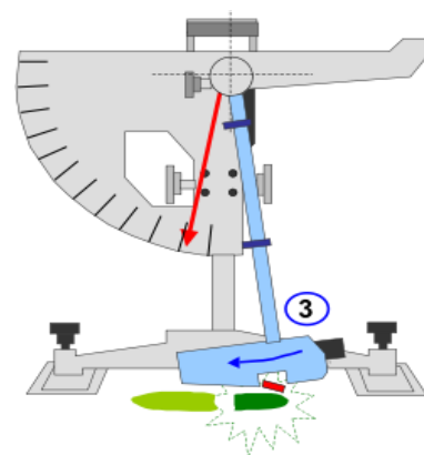
مرحله ۳: تماس قطعه لاستیکی آونگ با سطح پوشش (شبهه به پاشنه کفش) و حرکت نشانه‌گر بر روی سطح مدرج، همزمان با حرکت آونگ
